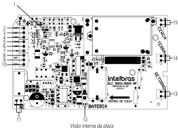
Visão interna da placa
